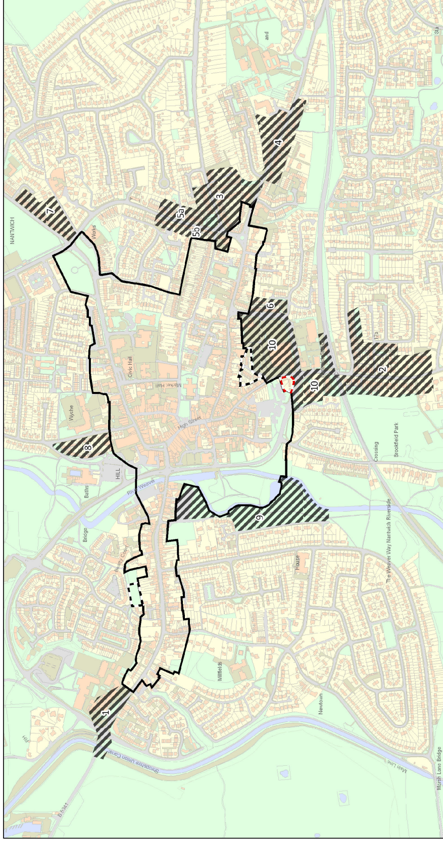
Map 1
